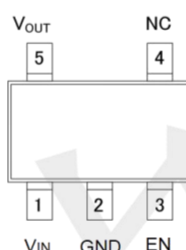
SOT23-5
