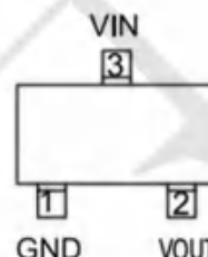
SOT23-3L & SOT23
